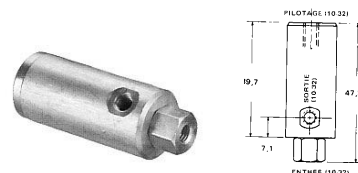
VALVE 2 voies à tiroir n/o commande par poussoir ,retour par ressort MAVO-2
