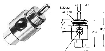
VALVE 2 VOIES à clapet n/f commande par poussoir retour par ressort MAV-2
