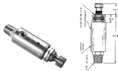
RÉGULATEUR DE PRESSION AVEC ORIFICE DE DÉCHARGE MAR-1P
