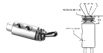
VALVE 3 voies à clapet commande par poussoir, retour par ressort MJV-3 n/f MJVO-3 n/0
