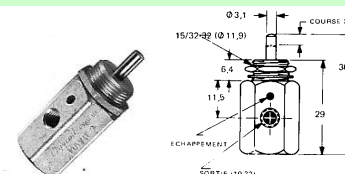
VALVE 3 voies à tiroir n/o commande par poussoir retour par ressort MAVO-3
