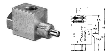
VALVE 2 voies à clapet commande par poussoir, retour par ressort MJV-2 =ref 6-030 n/f MJVO-2 n/0
