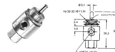
VALVE 3 voies à clapet n/f commande par poussoir retour par ressort MAV-3
