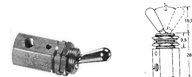
VALVES 3 VOIES à tiroir commande par levier 2 positions .pour air avec échappement TV-3S
