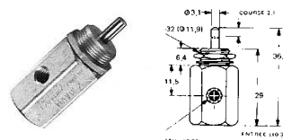
VALVE 2 voies à tiroir n/o commande par poussoir ,retour par ressort MAVO-2
