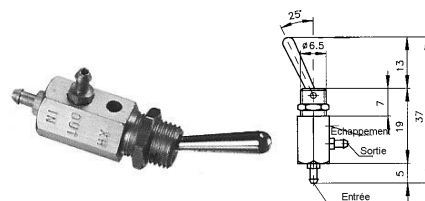
VALVE MINIATURE 3 VOIES à TIROIR N/F à levier 2 positions SMTV-3
