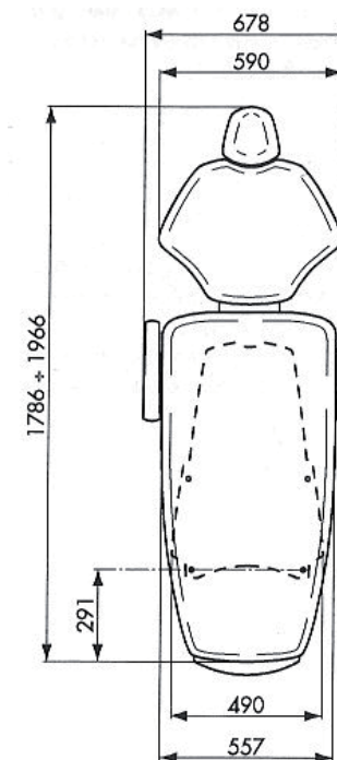
Dimensions PRO-04 et ORTHO-04
