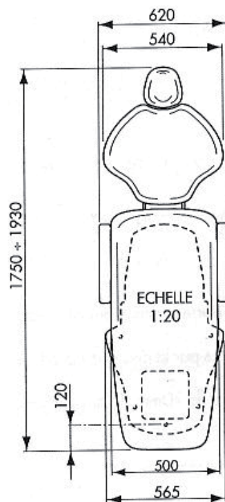
Dimensions PRO-03 et ORTHO-03
