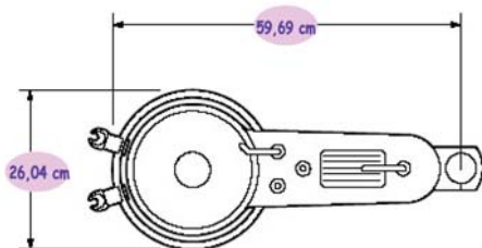
DIM Crachoir REF 1-566 new et 1-567 new
